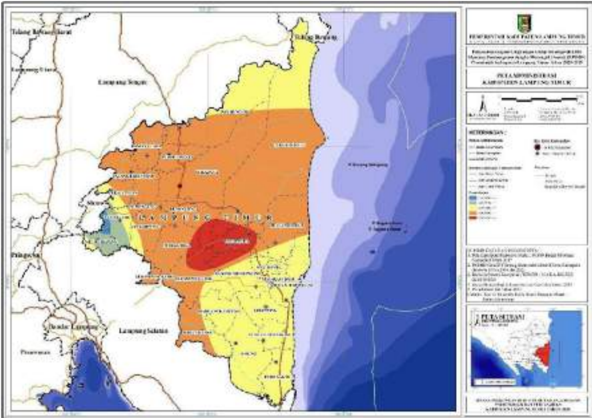
Gambar 2.18 Peta Curah Hujan Kabupaten Lampung Timur
