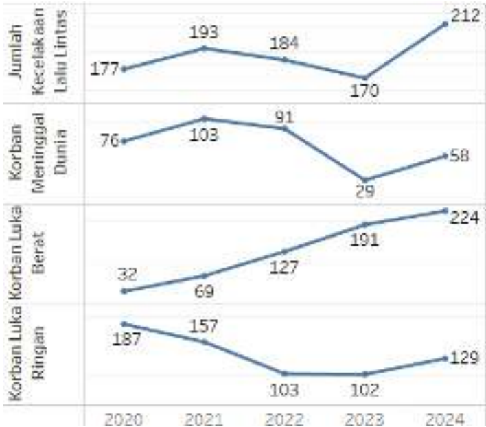
Grafik 2.76 Jumlah Kecelakaan Lalu Lintas dan Jumlah Korban Kecelakaan Kabupaten Lampung Timur
